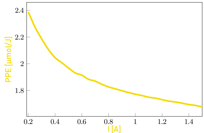
Photoneneffizienz vs. Strom
